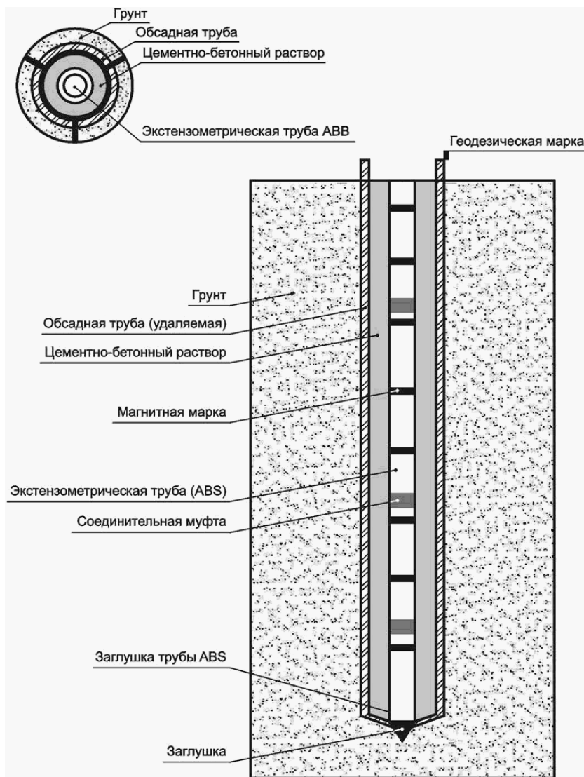
Рисунок Д.2. Схема экстензометрической наблюдательной скважины
