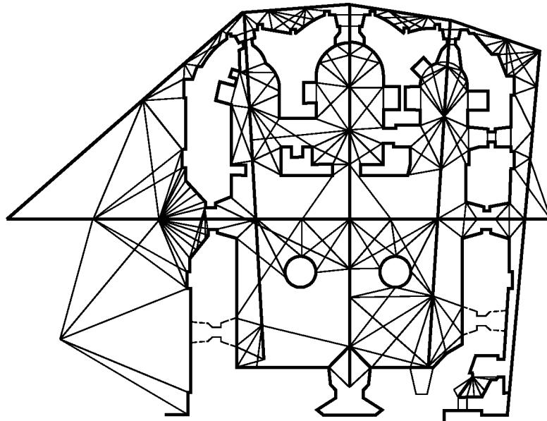
Рисунок Б.2 - Схема обмера плана с причалками
