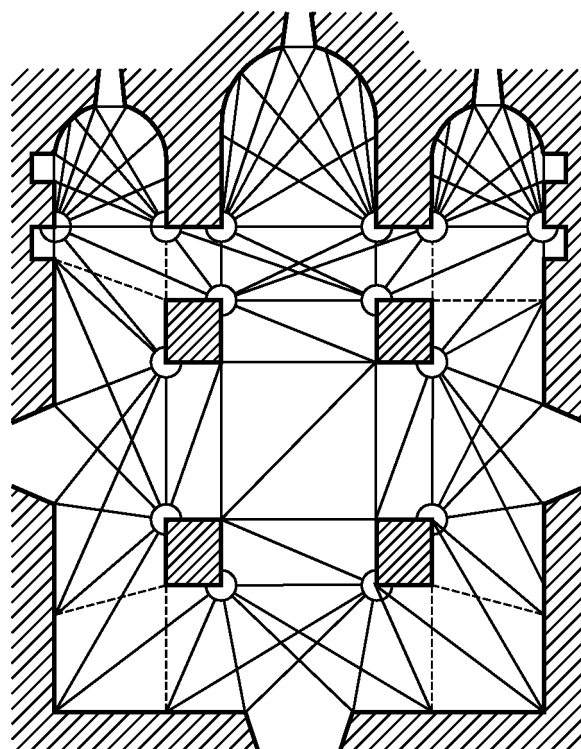
Рисунок Б.1 - Схема обмера плана методом триангуляции
